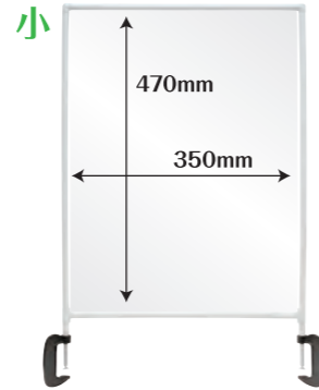
本体フレーム&フィルム サイズ:小 設置方法:Cクランプ シートサイズ: W350×H470mm
